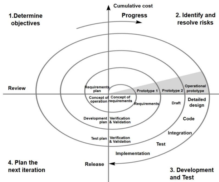
ภาพที่ 1.6 แบบจำลอง Evolution Model (Iterative)
